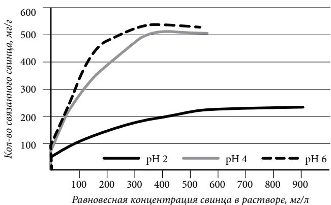
Рис. 4. Изотерма сорбции свинца образцом № 3 при pH 2–6.
