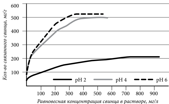
Рис. 3. Изотерма сорбции свинца образцом № 2 при pH 2–6.
